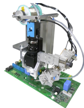
Lötkopf: Laser mit integrierter Kamera und Lotvorschub
